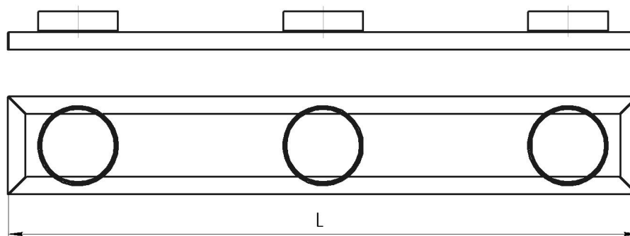
Рис.1 Подставка ДЖЕТ.214.03.00.00
